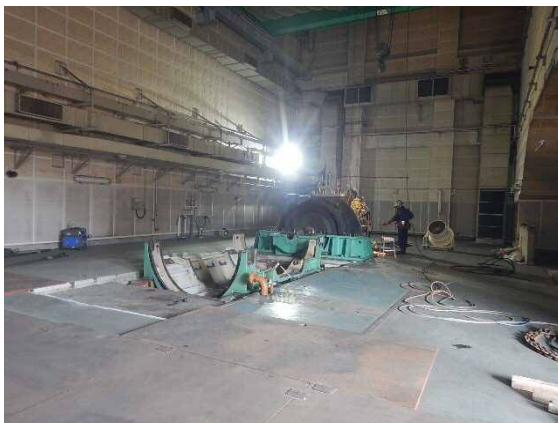
写真④ 発電機解体状況
