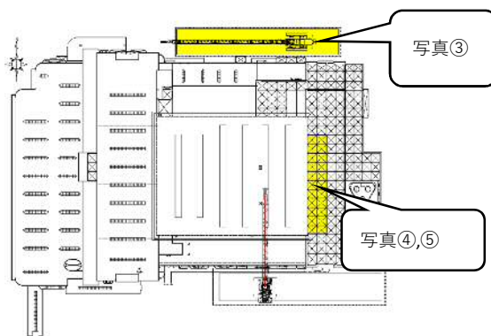
写真③ 北側クレーン状況
